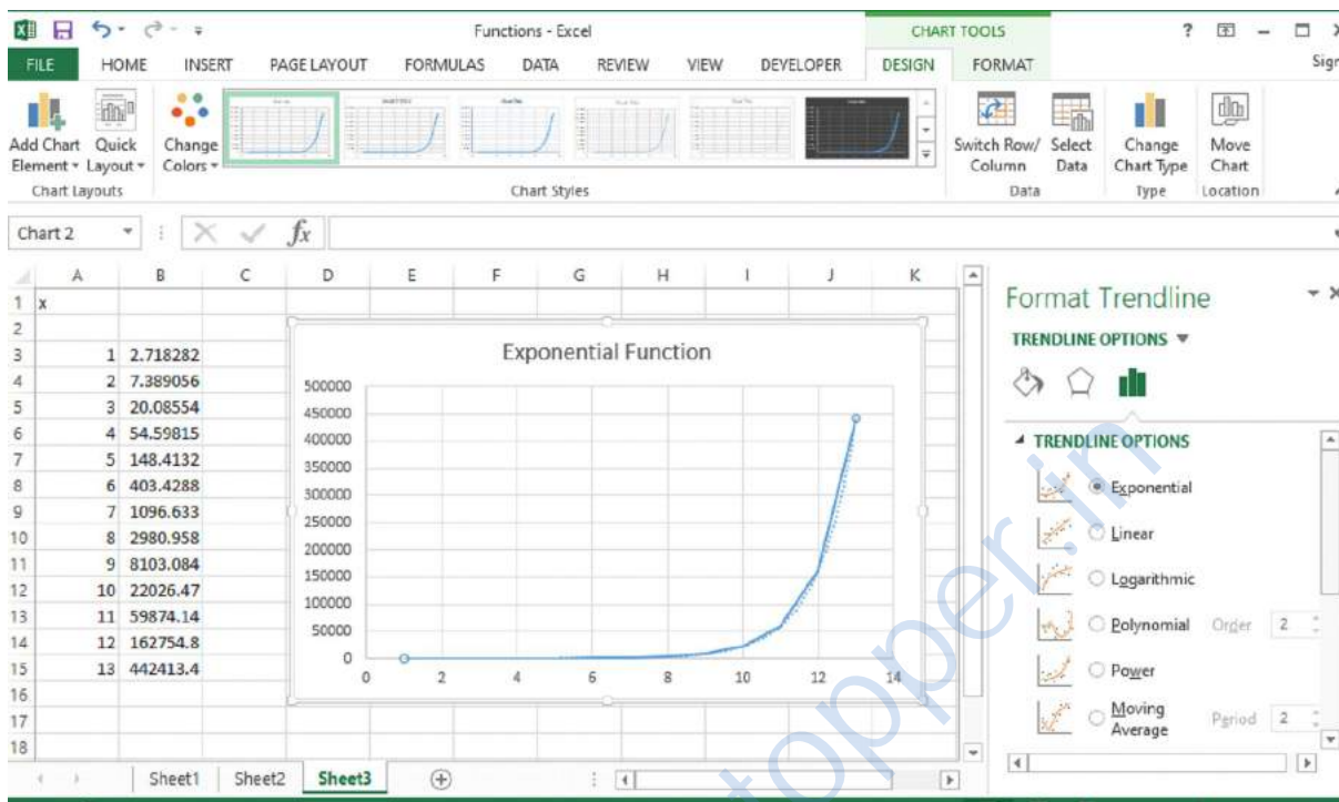
Fig 42: Exponential TRENDLINE
